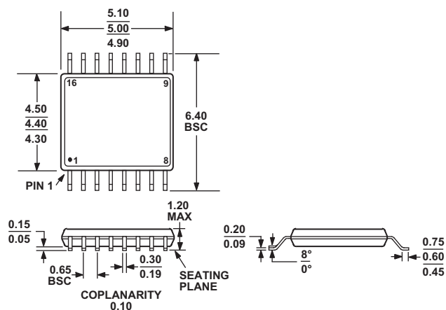
图22. 16引脚超薄紧缩小型封装[TSSOP] (RU-16) 尺寸单位: mm
